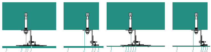
Epsilon T - Uñas ocultas Epsilon L - Uñas ocultas Epsilon T - Uñas vistas Epsilon L - Uñas vistas
